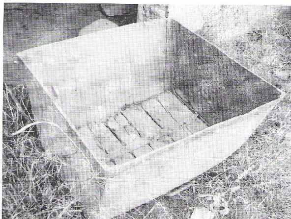
Canasta del viejo cable aéreo que se puede encontrar en Carabinera.
